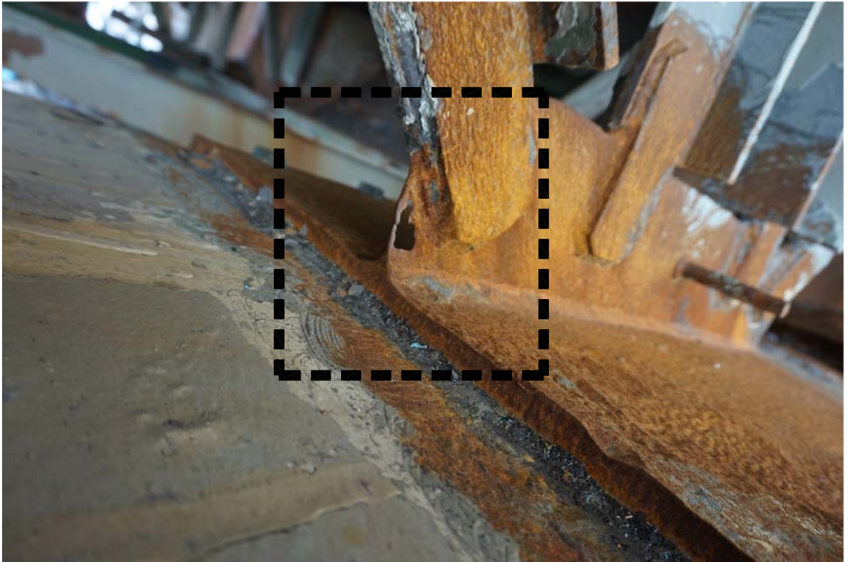
ESEMPIO TIPO: RIDUZIONE DELLO SPESSORE FAZZOLETTO VERTICALE SP. 12 mm
